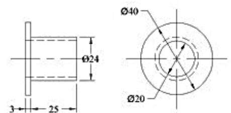
BUSH (BRZ.)
